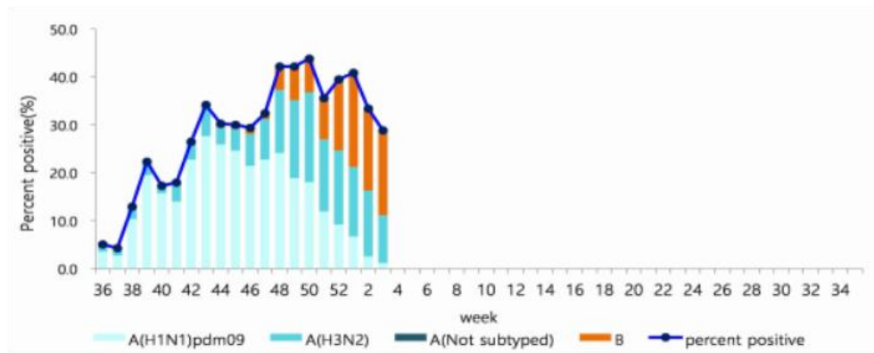
图 17 韩国流感毒株检测情况
